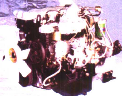
CA4118ZL 型增压中冷柴油机
