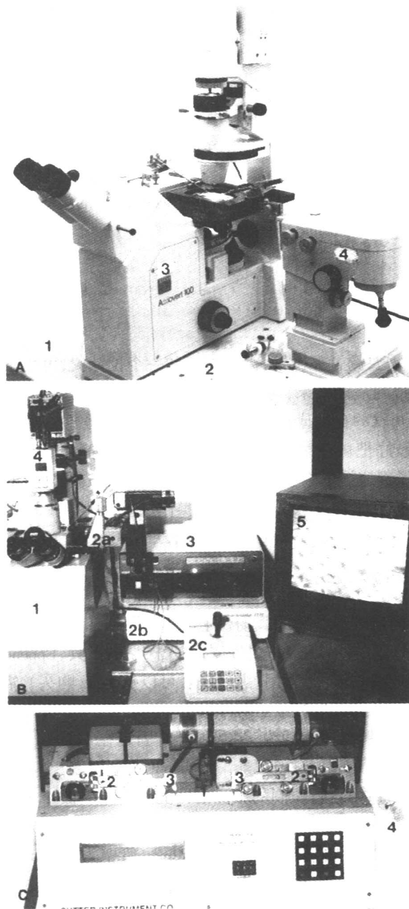
图 1.1A-C 安装好的手动与自动微注射设备(见材料部分)。A: 手动微注射设备的组成部分:1.防震桌;2. Leitz 重型底座;3. Zeiss Axiovert 倒置显微镜;4. 右手 Leitz 微操作仪。B: 自动微注射设备的组成部分:1. Zeiss 倒置显微镜;2. Eppendorf 自动微操作仪(5171 型):2a 为微操作部分,上面有三个电动马达驱动的部分,可在 x、y、z 三个方向运动;2b 为电源部分;2c 微电脑部分,配有键盘和操作杆;3. Eppendorf 微注射器(5242 型);4. 电视摄像机;5. 电视监视器,显示出盖玻片上需要注射的细胞,显示在右侧的微注射针头,指向屏幕中心。C: Sutter Instrument 产水平拉针仪(P-87 型) 1.加热丝固定器;2. 左右滑夹;3. 夹子;4. 玻璃毛细管。
