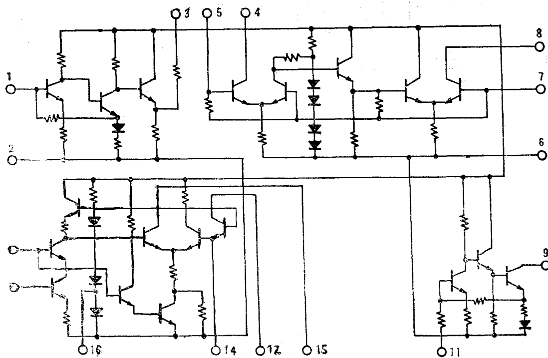
图5—1 AN217P等效电路
