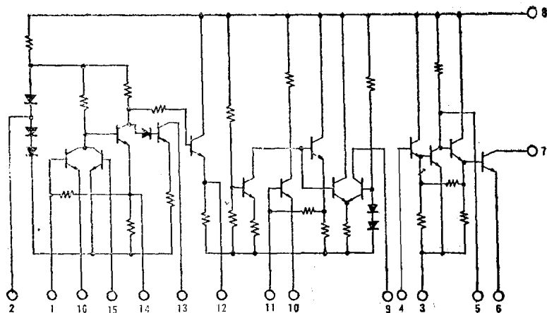
图6-1 AN253P 等效电路
