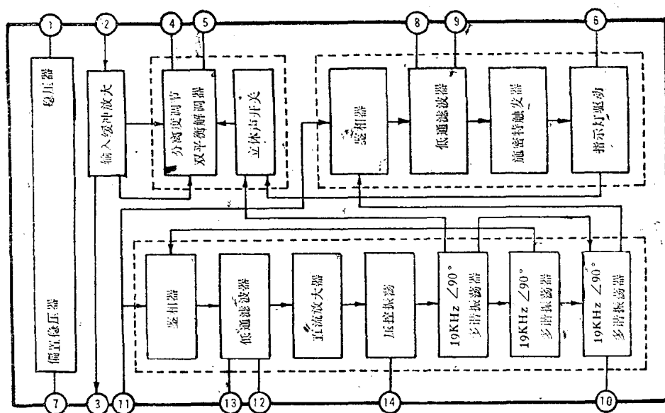
图3—1 AN115 方框电路
