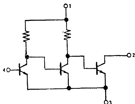
图1—1 OM200等效电路
