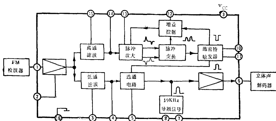
图2—1 AN101方框电路图
