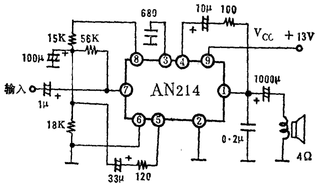
图4-2 AN214典型应用电路
