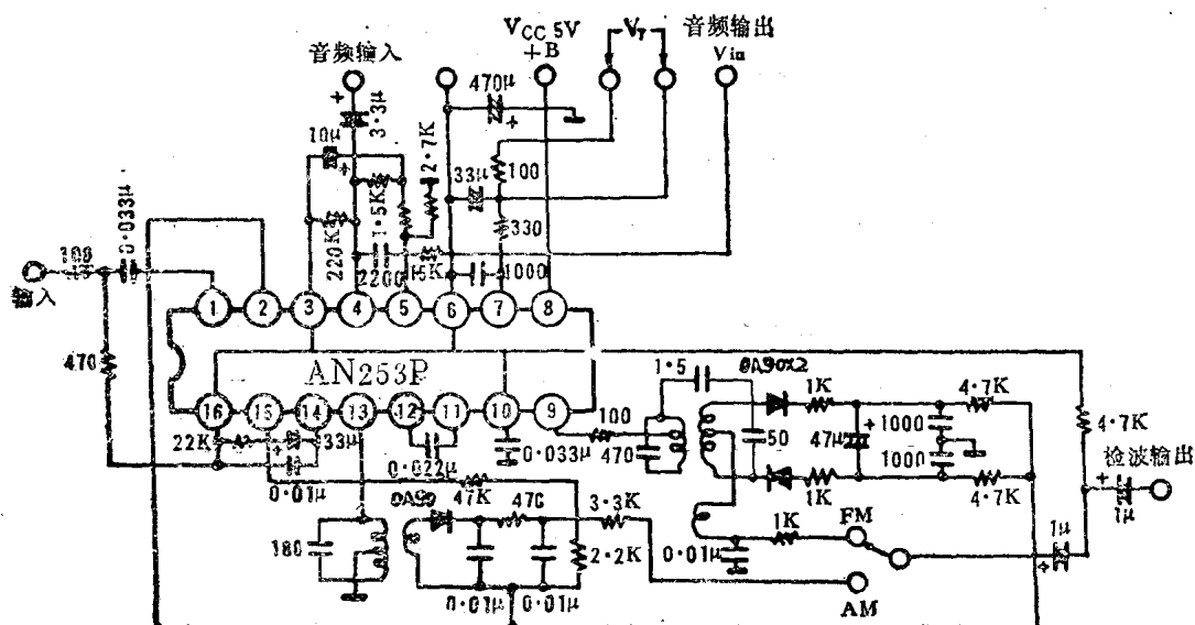
图6-2 AN253P典型应用电路
