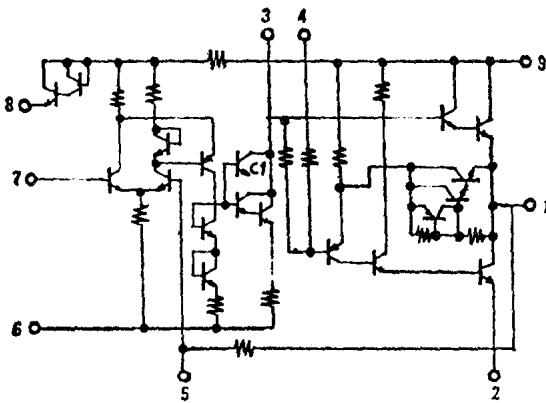
图4-1 AN214等效电路
