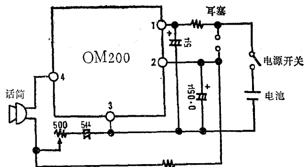
图1—2 OM200典型应用电路
