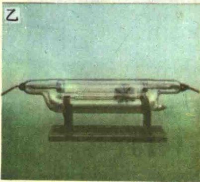
图5 阴极射线管
