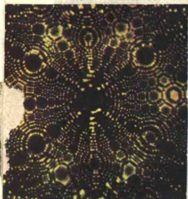
图1 钨原子
