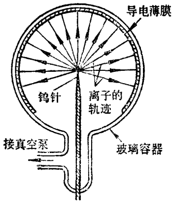
图 1-2 离子显微镜的构造原理
