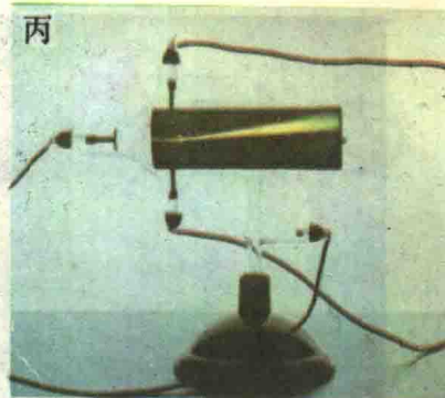
图4 辉光放电
