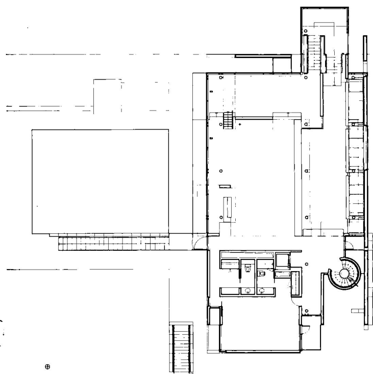
二层平面图
