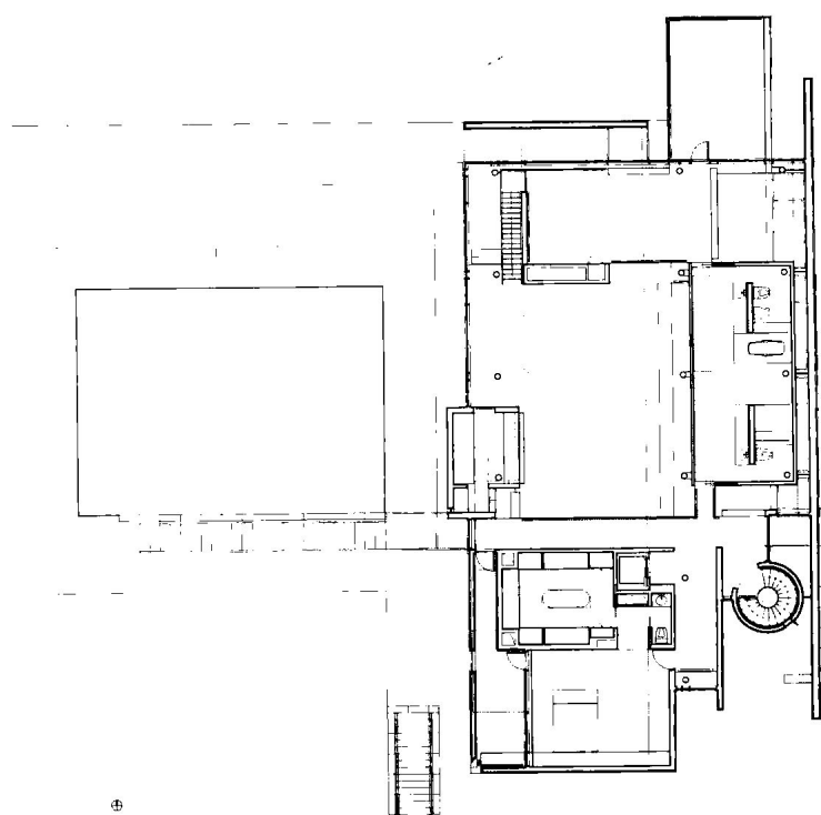
三层平面图
