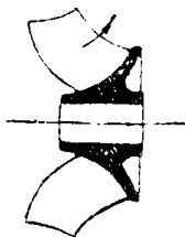
图 1-1-2 混流泵（混流式）叶轮的类型
