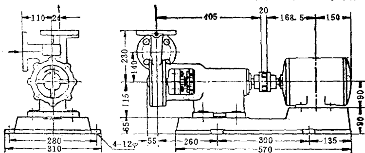
图 1-1-7 单级旋涡泵外形尺寸图
