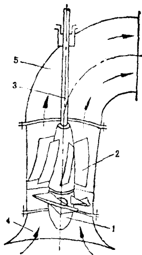
图 1-1-6 轴流泵的构造
