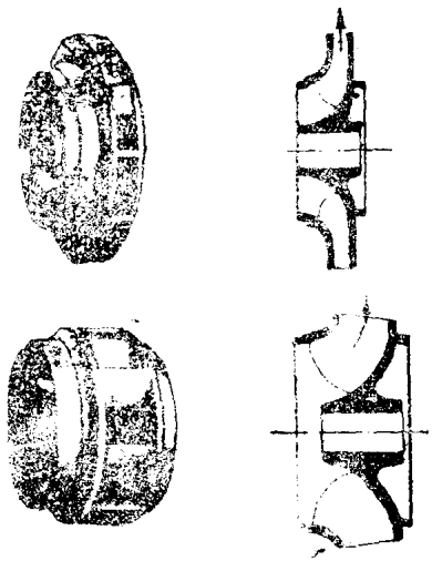
图 1-1-1 离心泵 (径流式)叶轮的类型
