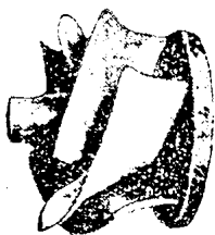
图 1-1-2 混流泵（混流式）叶轮的类型
