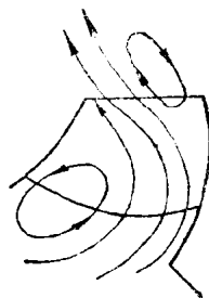
图 1-1-3 混流泵叶轮内的旋涡
