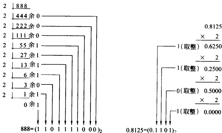
图 1-2 十进制数与二进制数转换
