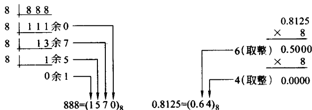
图 1-3 十进制数与八进制数转换
