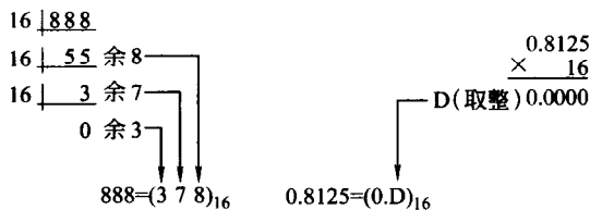
图 1-4 十进制数与十六进制数转换
