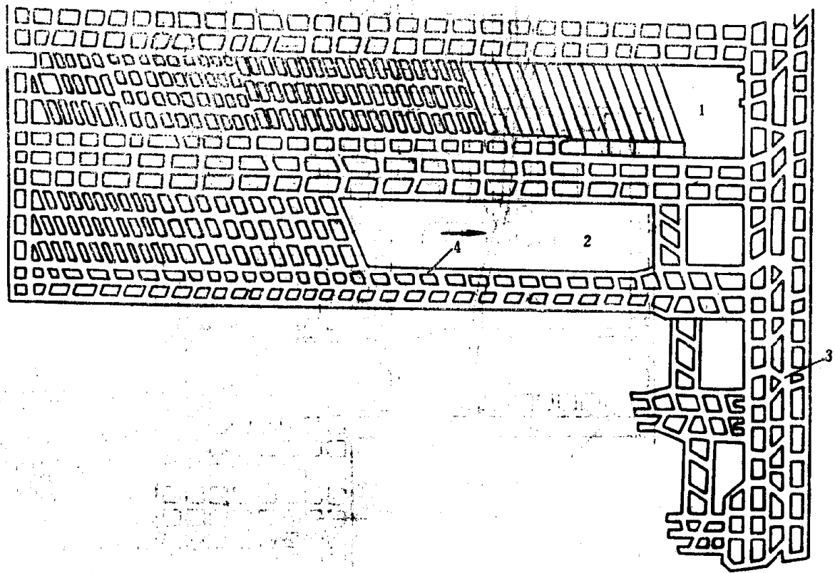
图2-7 在区段平巷一侧布置煤房
