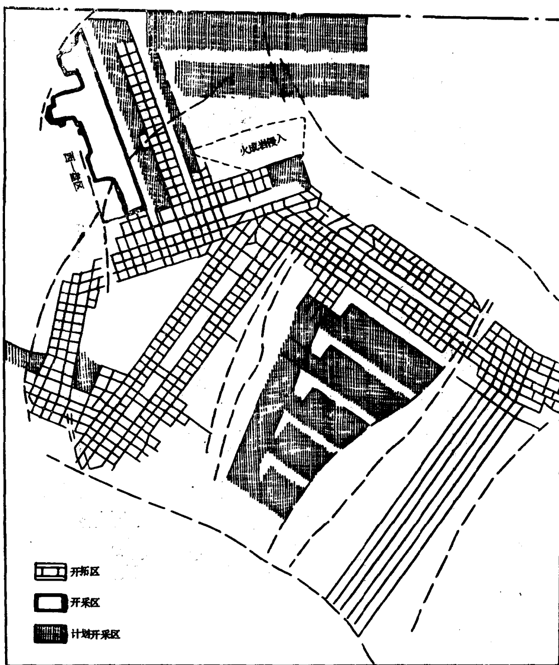
图 2-9 澳大利亚里水矿区库克矿开拓布置实例
