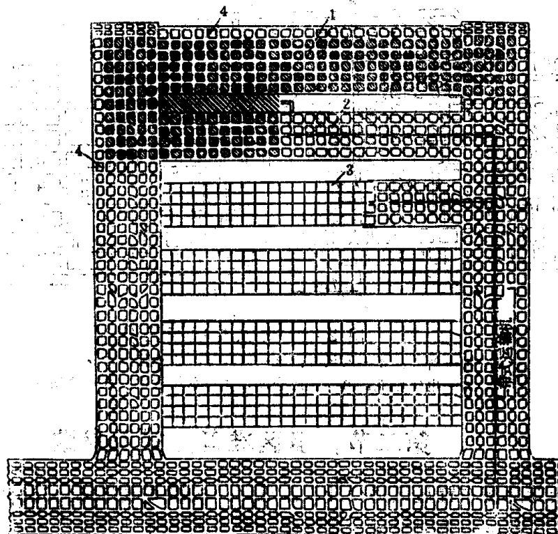
图 2-6 四边先用平巷圈定的盘区准备方式→
