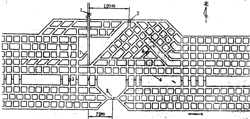
图2-4 井底巷道布置图
