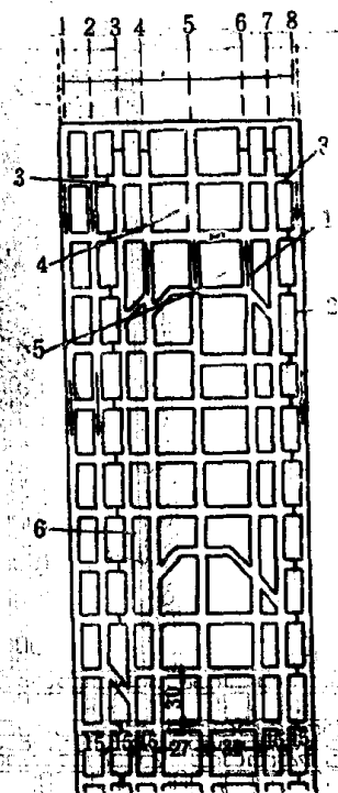
图2-3 根据压力拱理论进行平巷布置设计
