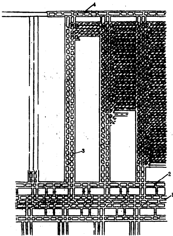
图 2-5 美国奥尔德·本公司的盘区准备方式
