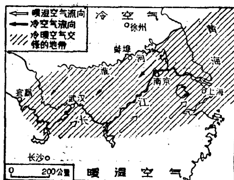
梅雨形成示意图
