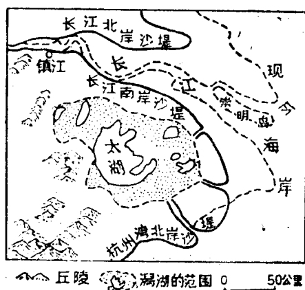
长江三角洲形成示意图
