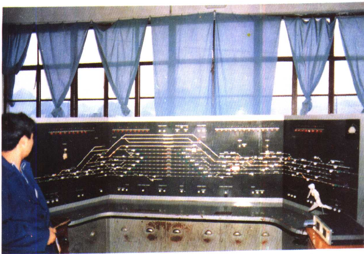
六盘水站行车集中控制台
