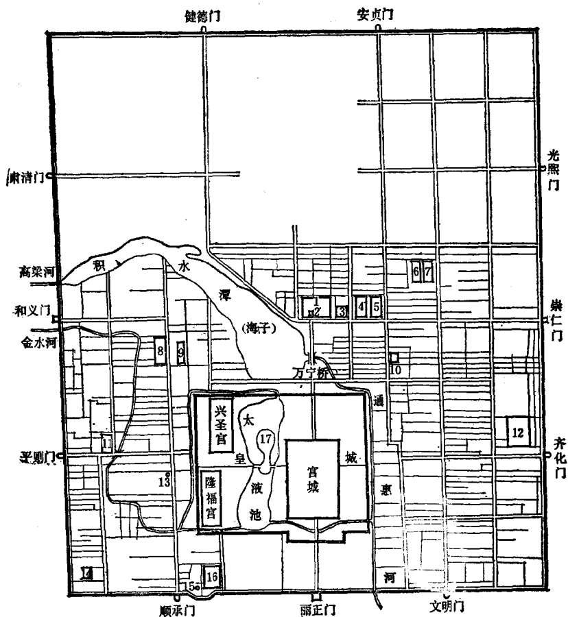
图 1-2 元大都图（摹自《考古》，72年1期）
