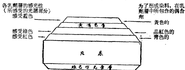
图一：彩色多層膠片的結構圖
