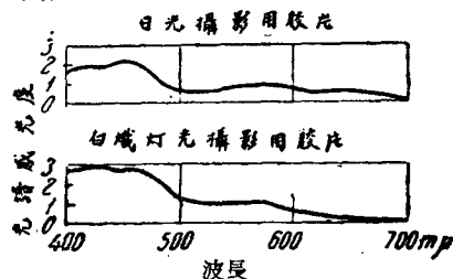
图五：白光和白熾灯光用彩色底片的光譜感光性
