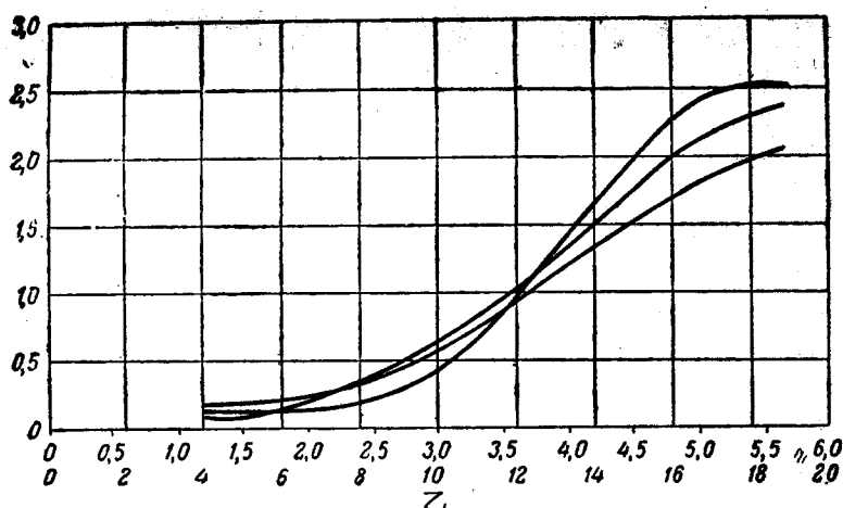
图六：多層彩色底片的特性曲綫
