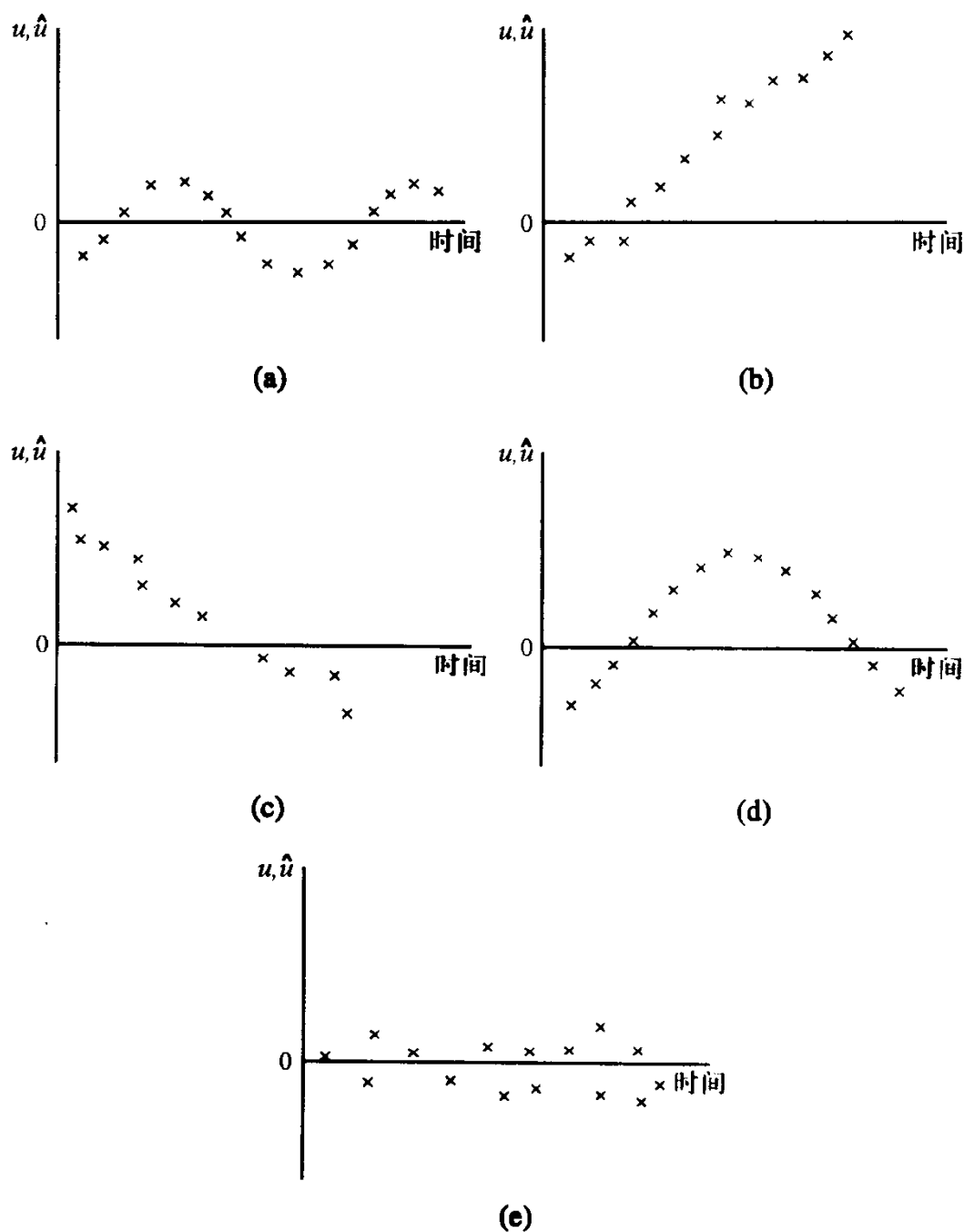
图 12.1 自相关模式
