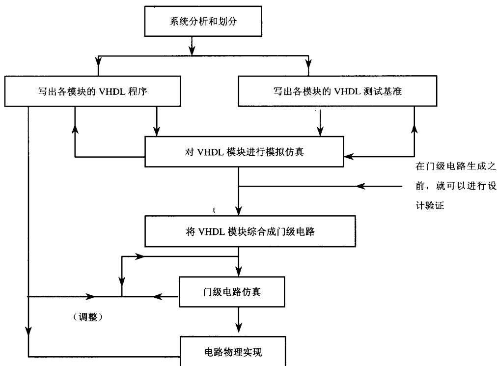
图 1.2 VHDL 设计流程
