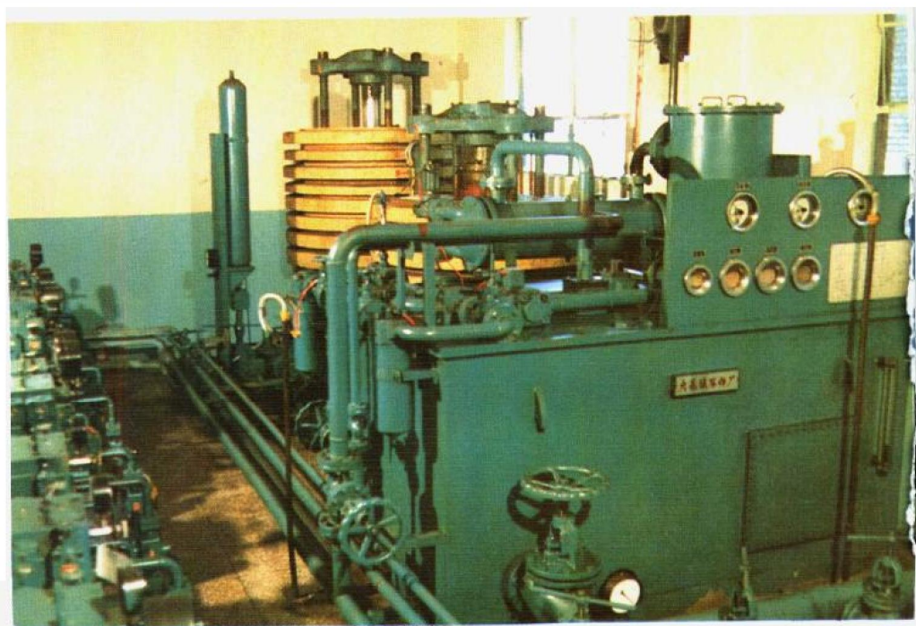
▶ 大连液压件厂研制的 的线材轧机大型成套液 压系统
