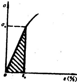
图1-1-3 弹性比功
