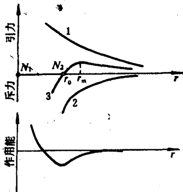
图1-1-1 双原子模型 1—引力曲线；2—斥力曲线；3—合力曲线。
