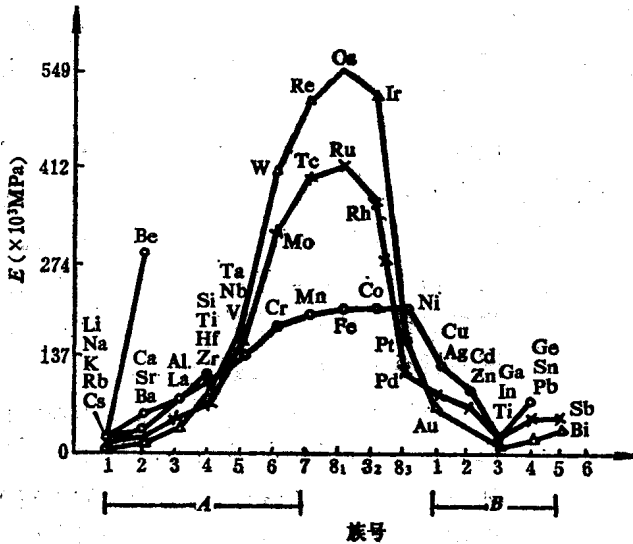
图1-1-4 金属元素弹性模量的周期变化
