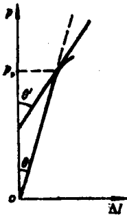
图1-1-2 比例极限 \sigma_p 的确定
