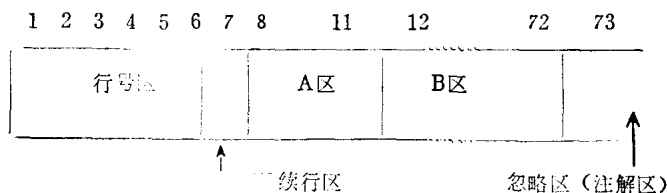
图 2.1 MS-COBOL源程序行格式
