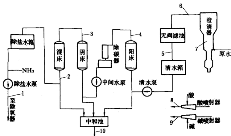
图 0-3 水处理系统化学监控采样点
