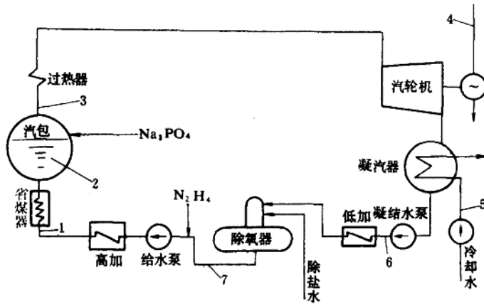
图 0-2 中等容量机组的水汽循环系统化学监控采样点
