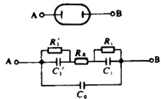
图 1-1 电导池的交流等效电路
