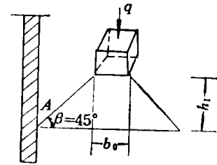
图 1-1-10 柱形基础对井颈产生的侧压力图
