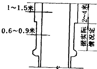
图 1-1-2 型式 I
