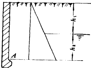
图 1-1-8 浸水砂土层侧压力图
