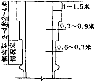
图 1-1-4 型式Ⅲ
