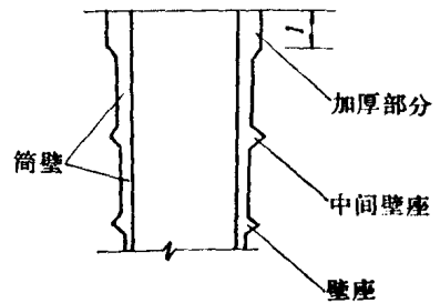
图 1-1-1 井颈的组成
