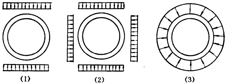
图 1-1-11 侧压力的种类
