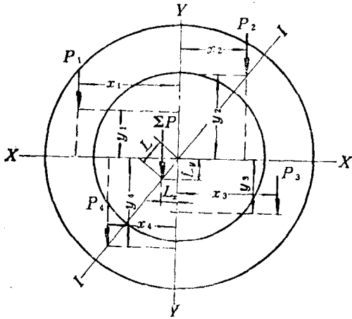
图 1-1-15 偏心作用时合力中心计算图
