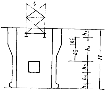
图 1-1-7 确定井颈最小高度示意图
