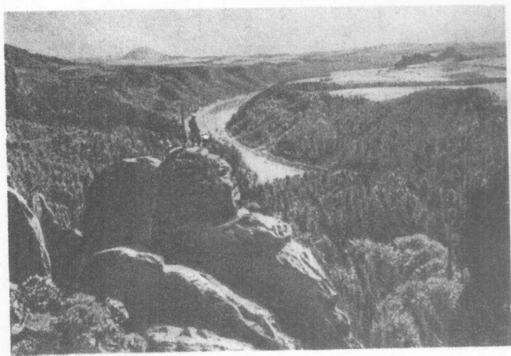
捷琴城区来北河河谷風景；前景是由于砂岩風化所形成的悬岩。
