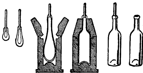
圖 5. 怎樣製玻璃瓶
