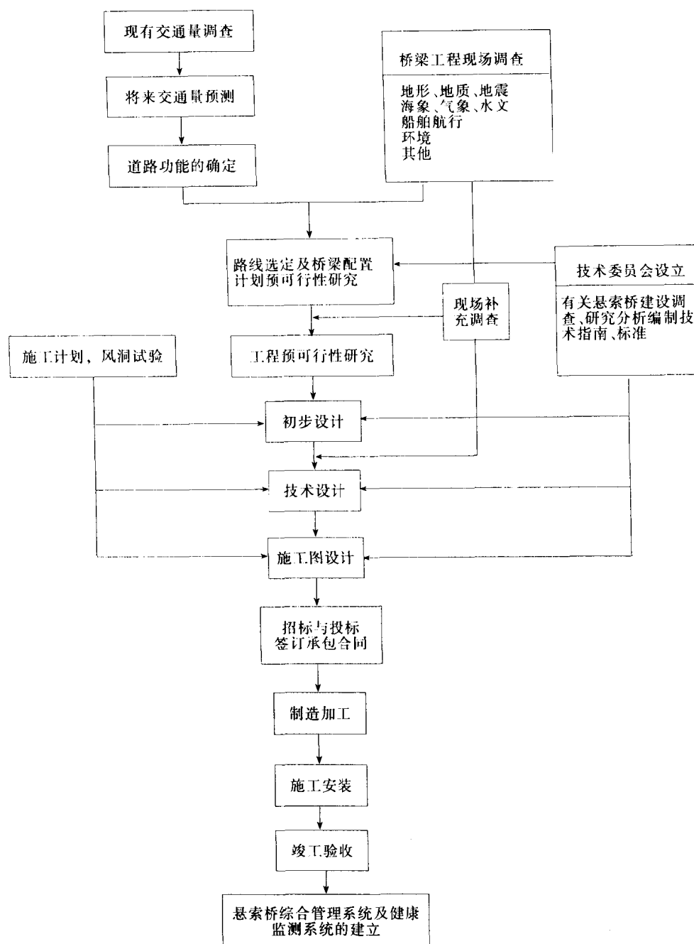
图 1-1-1 悬索桥建设的工作程序
