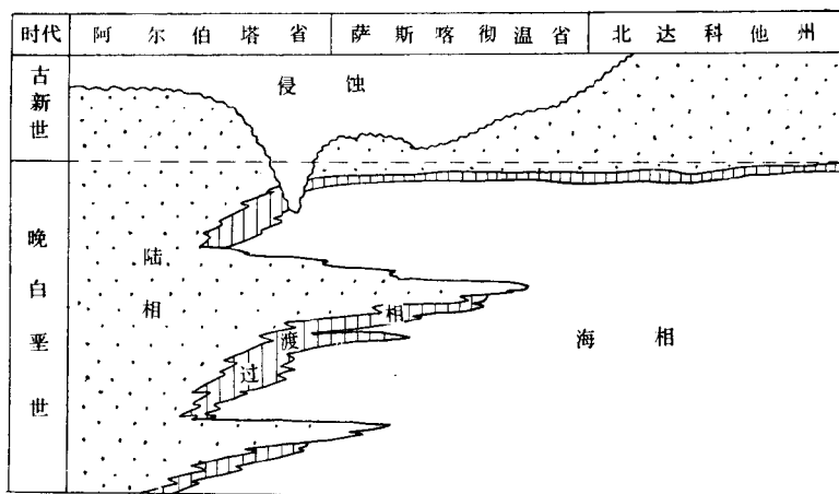
图 3 (据 Caldwell 1968简化)
