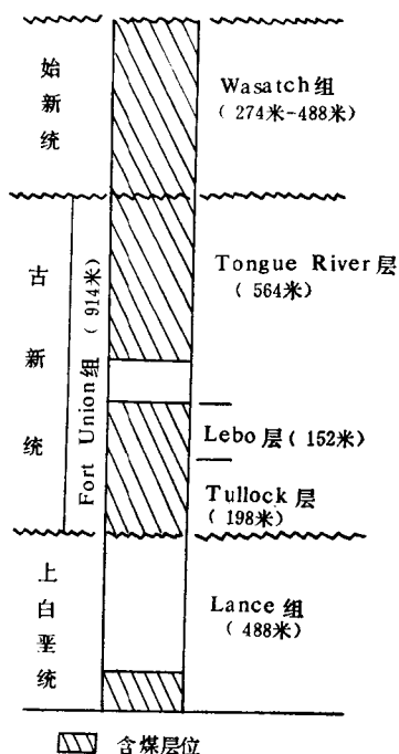
图 4 泡德河盆地的含煤组 (据 G. B. Gloss)
