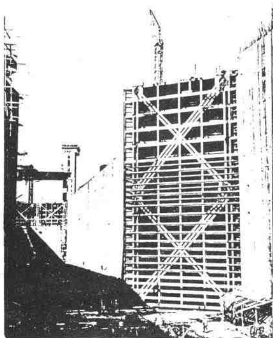
图 0-2 葛洲坝 2 号船闸安装时的人字钢闸门
