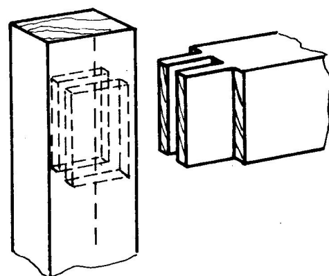
双榫结合
