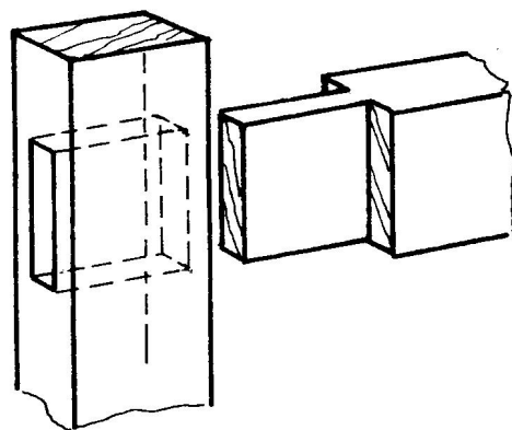
贯通榫结合
