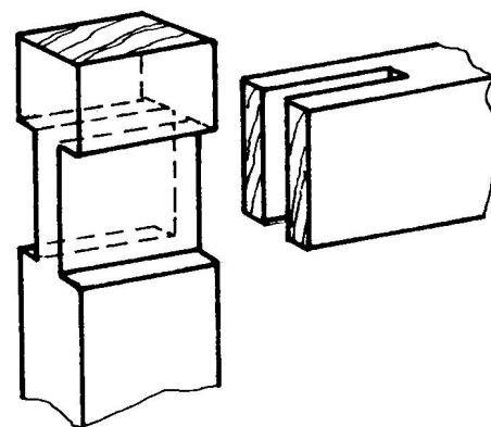
夹皮榫结合
