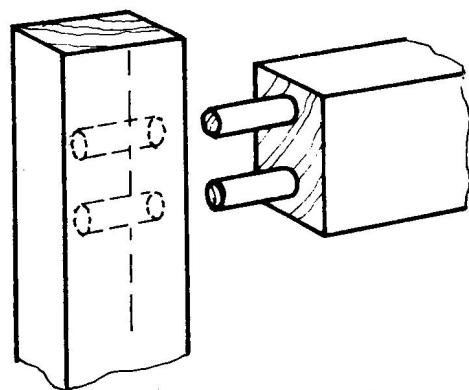
圆棒榫结合
