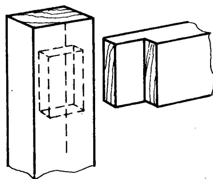
单肩榫结合
