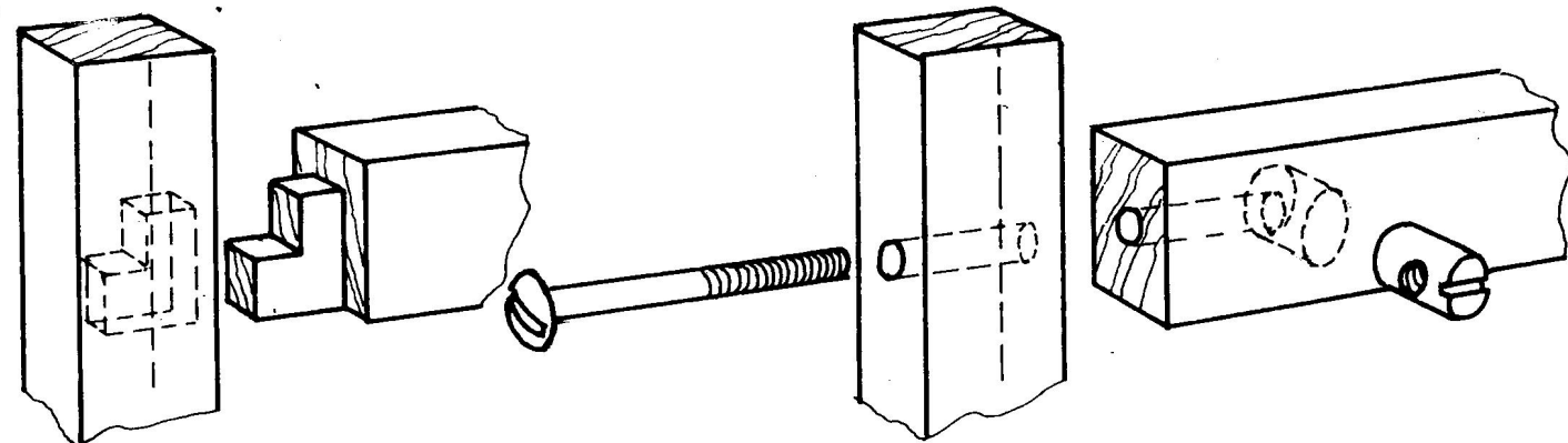
金属圆柱螺母结合
