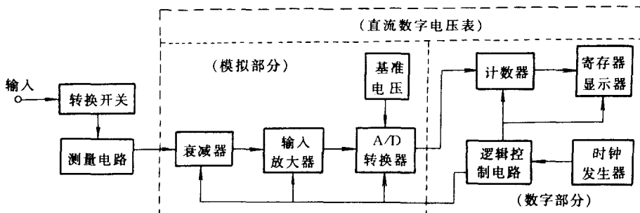
图 1-1 袖珍数字万用表电路结构
