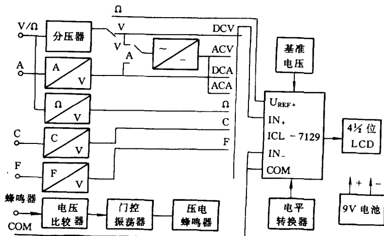
图 1-4 DT-980 袖珍数字万用表原理方框图
