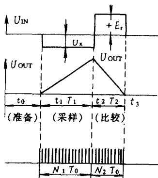
图 1-3 工作波形
