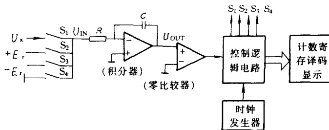
图 1-2 双斜积分式 A/D 转换器原理
