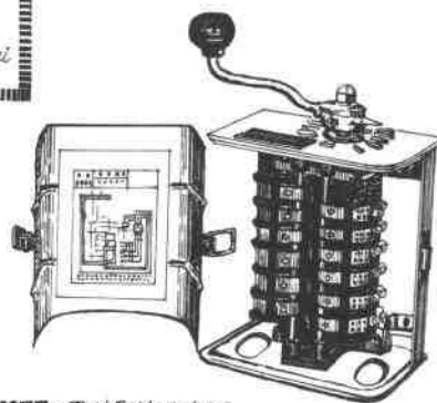
KTJ6系列凸轮控制器
