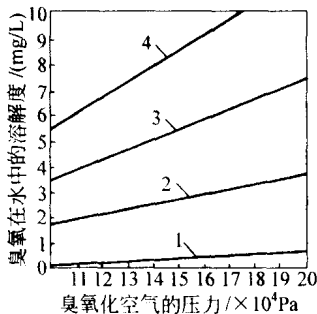
图 1-1 压力对臭氧溶解度的影响 1—1gO 3 /m 3 空气；2—5gO 3 /m 3 空气； 3—10gO 3 /m 3 空气；4—15gO 3 /m 3 空气
