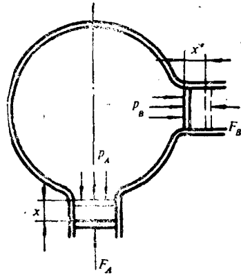
图 2.1 液体压力传递示意图
