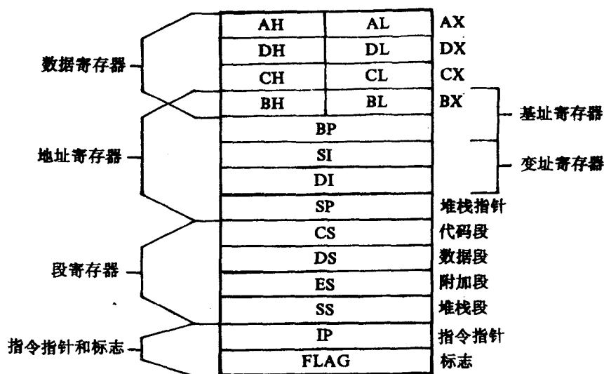
图 1.2 8088 CPU 内部寄存器
