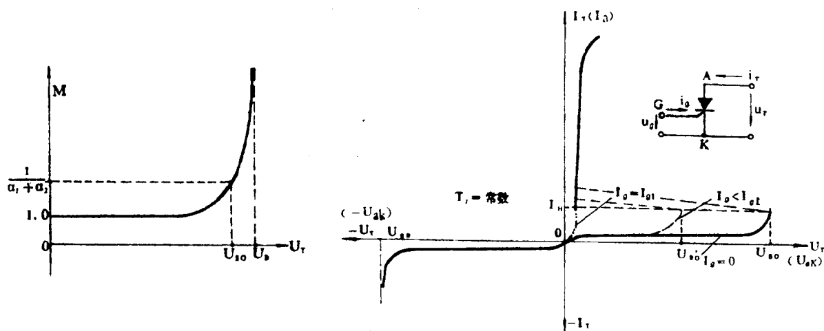
图1-2 倍增因数与阻断电压的关系
