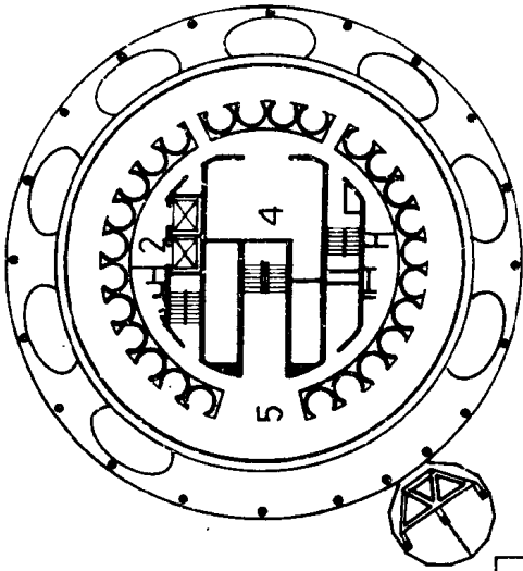
主厅平面
