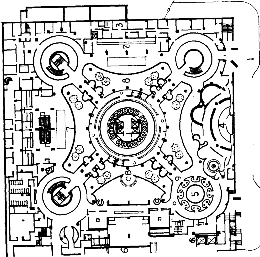
入口层平面
