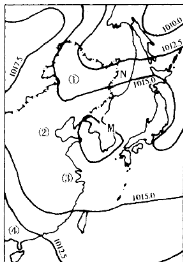
某时海平面平均气压(单位: hPa)
