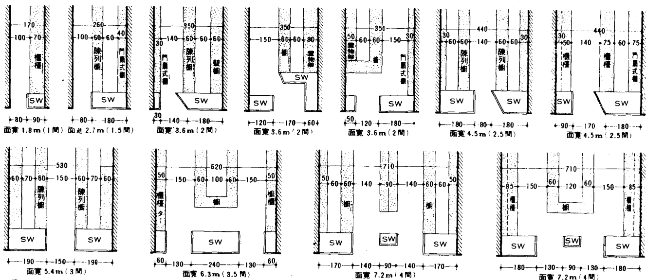
a 直接樓梯
