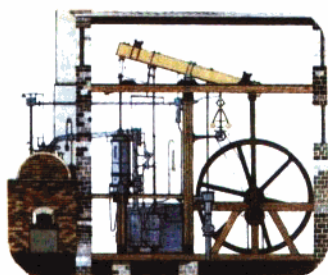
蒸汽机
