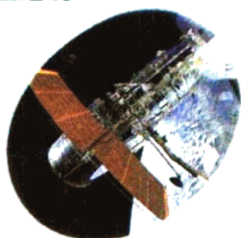
哈勃望远镜
