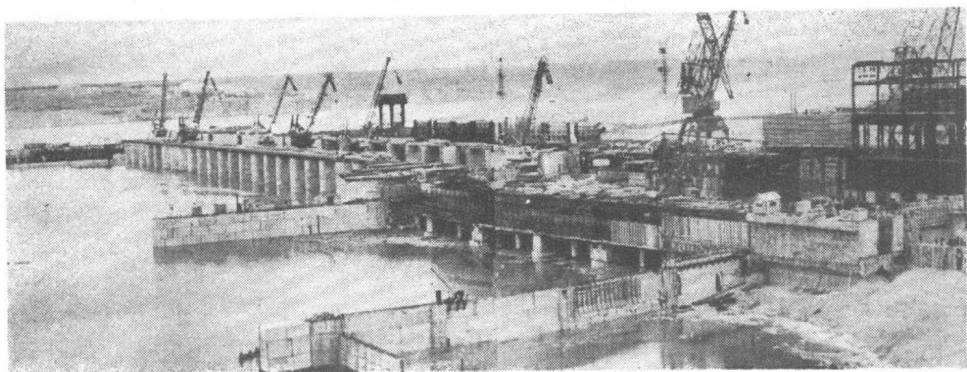
卡霍夫卡水電站溢洪壩建築工程。
