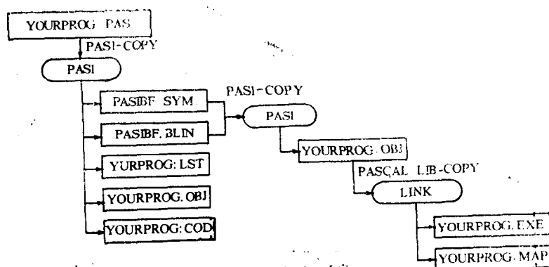
图 2.1 如何翻译你的程序
