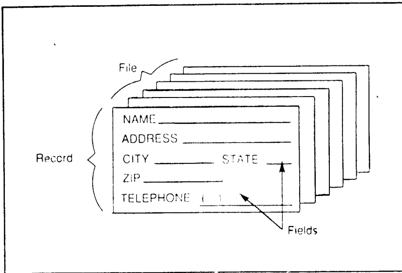
图 I-1 数据库术语
