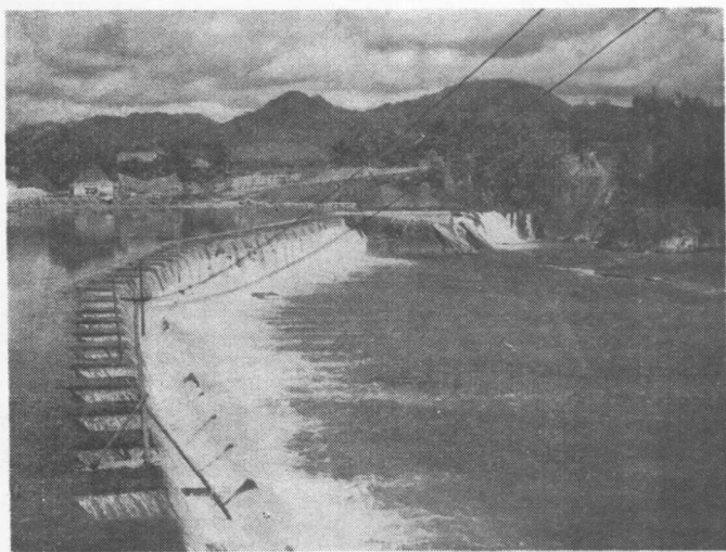
越南沛上水利工程(越南修復最大水利工程之一)
