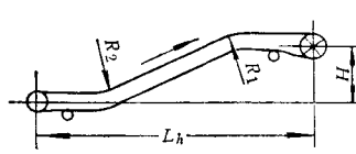
图6-1-5 水平-倾斜-水平输送机
