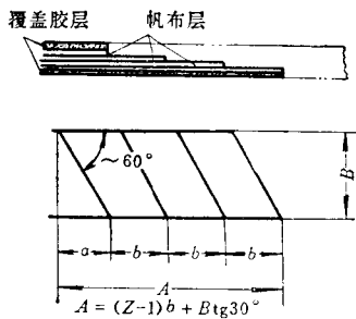
图6-1-10 硫化接头裁剖图
