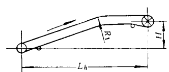
图6-1-3 倾斜-水平输送机
