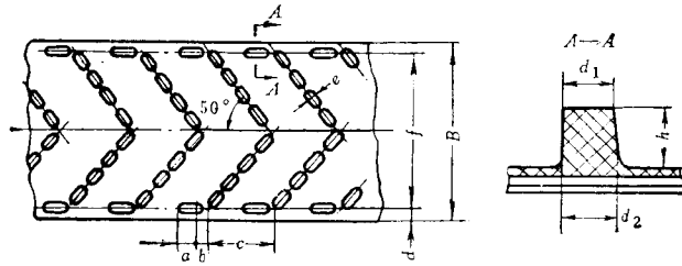
图6-1-8 条状花纹胶带示意图
