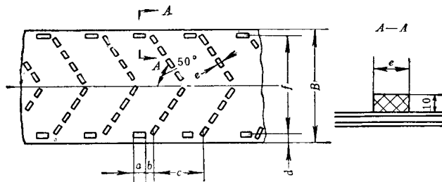
图6-1-9 花纹塑料带示意图
