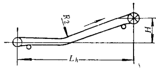
图6-1-4 水平-倾斜输送机
