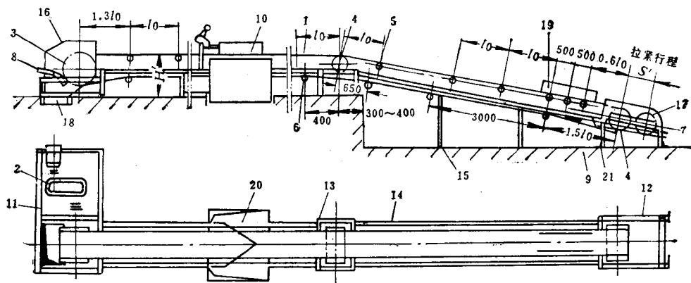
图6-1-7 TD型带式输送机的部件组成示例
