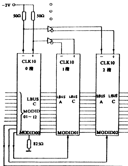
图 1 CLK10, MODID 和 LBUS 背板信号传输路径
