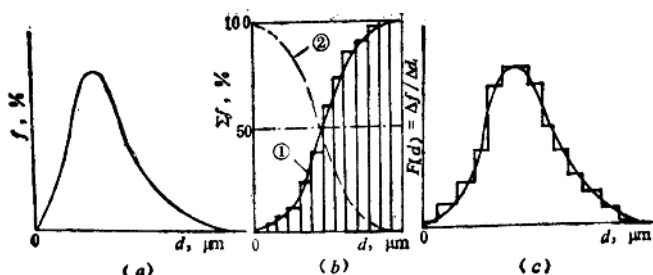
图 1-2 粒度分布曲线形态 (a) 粒度分布; (b) 累积分布; (c) 微分分布
