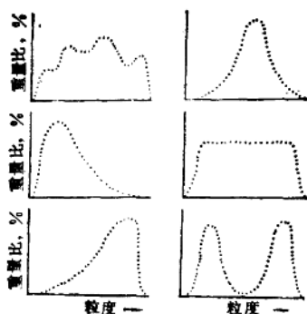
图 1-1 各种类型的粉末粒度分布
