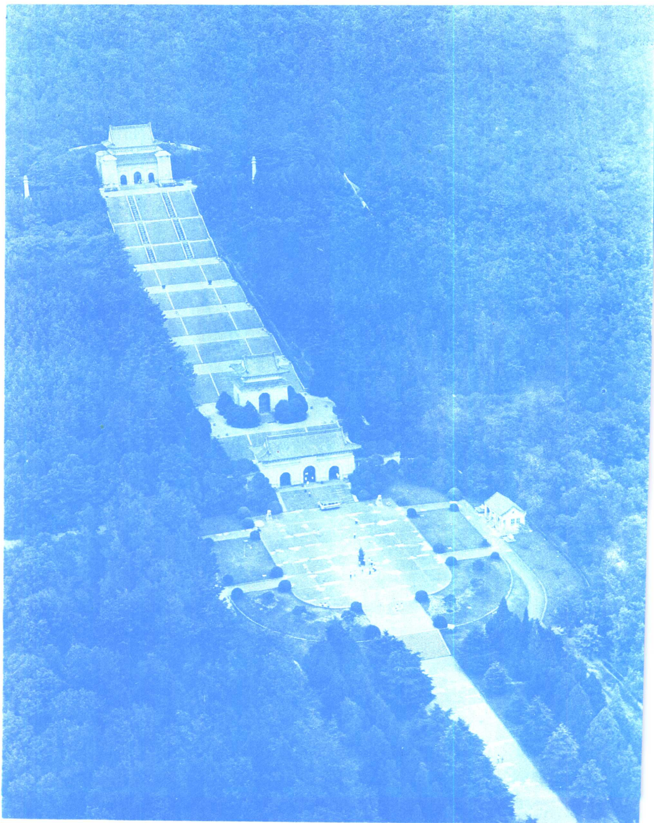
1 中山陵 南京 1926~1931 设计：吕彦直。陵墓总平面呈钟形，纵深700 m， 自南而北布置牌坊、墓道、陵门、碑亭、石阶、祭堂和墓室
