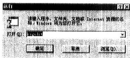
图 1-6 “运行”对话框
