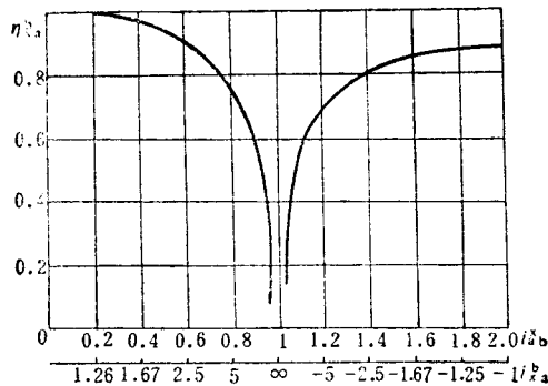
图 16-3 WW 型效率曲线 ( \varphi^x = 0.06 作出)
