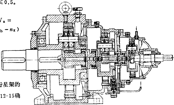
图 16-10 NGW型三级行星传动
