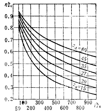
图 16-5 NGWN 型效率曲线 ( f = 0.12 , \mu = 0.006 作出)
