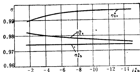
图 16-2 NGW及NW型效率曲线 ( \varphi^x = 0.025 作出)
