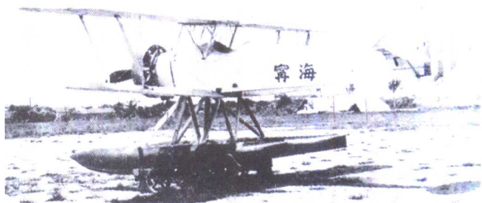
中国 1933 年制 造的“宁海” 号水上侦察机
