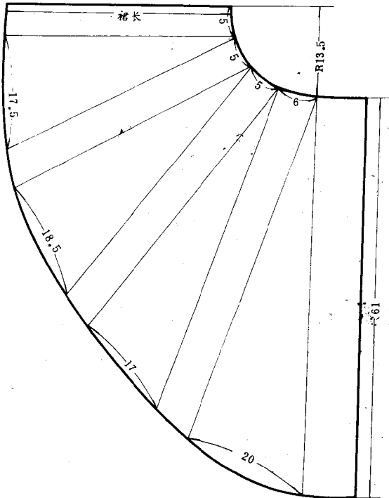
制图尺寸 单位: 厘米
