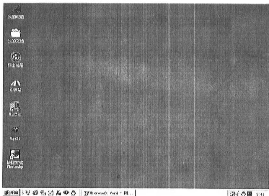
图 1.8 Windows 98 桌面
