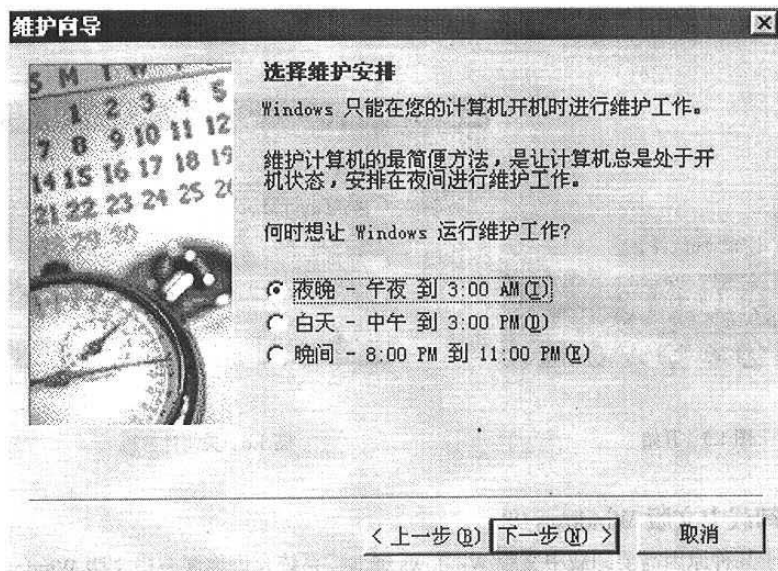
图 1.3 维护向导 (2)
