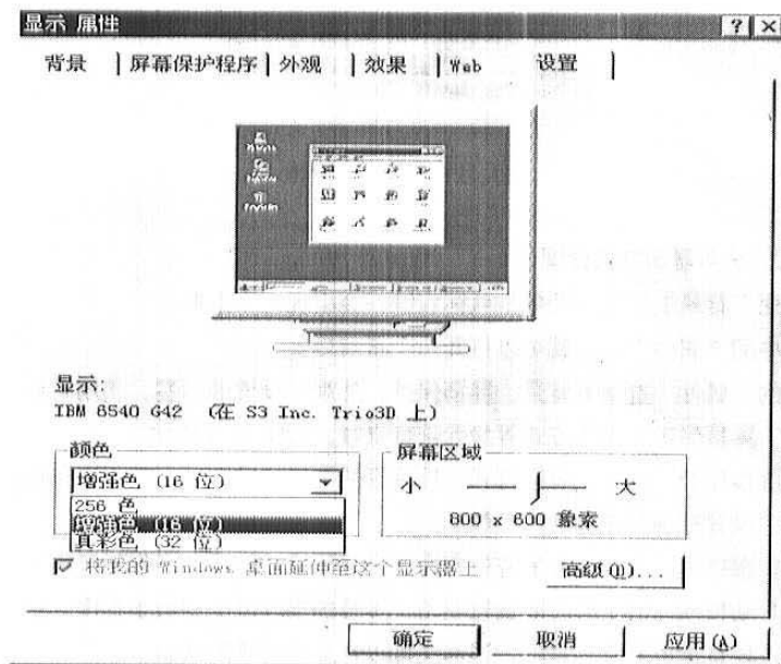
图 1.16 “设置”标签
