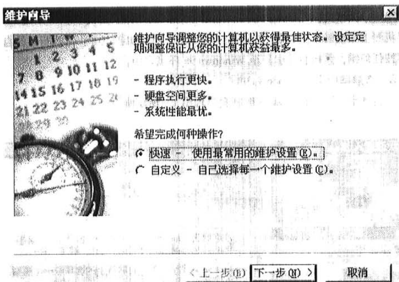
图 1.2 维护向导 (1)
