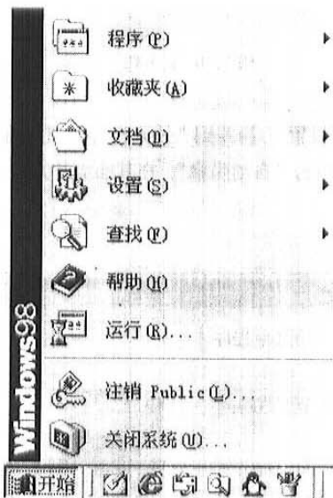
图 1.12 开始菜单
