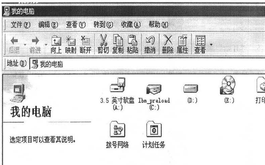
图 1.17 “我的电脑”
