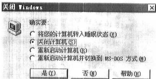
图 1.6 关闭计算机
