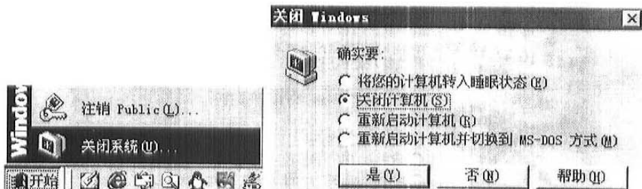
图 1.5 开始
