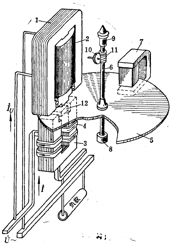
图 2-1 单相电度表的测量机构简图
