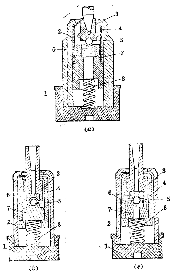
图 2-4 钢珠宝石轴承的三种基本类型 (a)正宝石轴承, (b)倒宝石轴承, (c)双宝石轴承 1—螺帽; 2—衬管; 3—轴承; 4—卡套; 5—钢珠; 6—宝石; 7—支承; 8—弹簧
