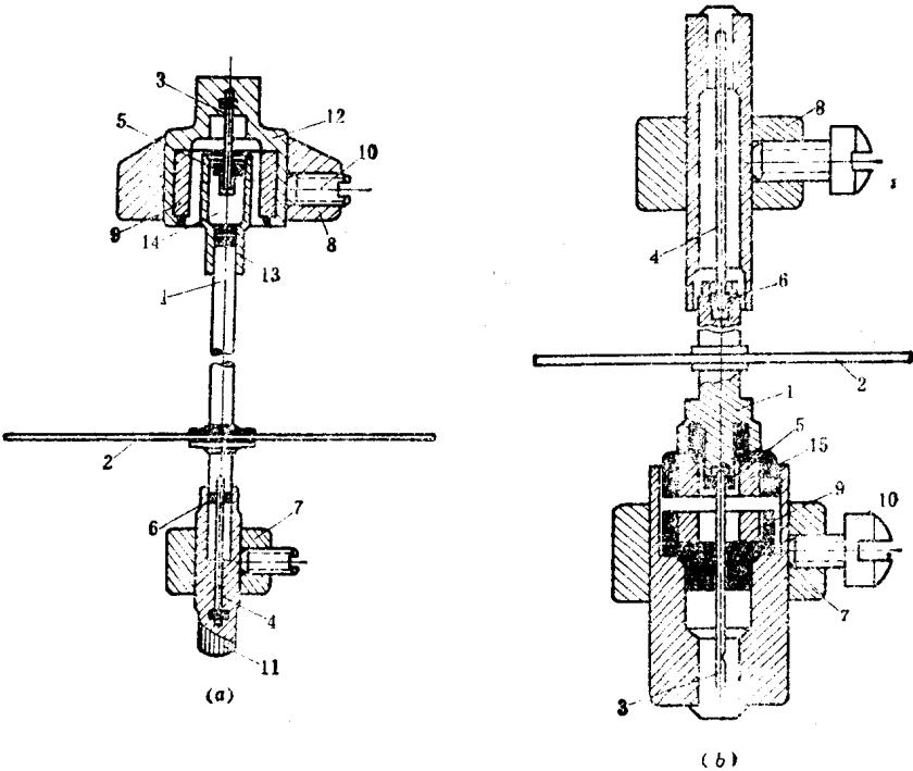
图 2-6 磁力轴承
