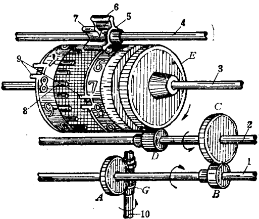
图 2-8 字轮式计度器 G—蜗杆，A—蜗轮；B、D—主动轮；C、E—从动轮，1~4—横轴，5—进位轮，6—长齿，7—短齿，8—稍齿，9—槽齿，10—转轴
