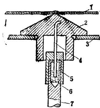
图 2-5 常用的一种上轴承结构 1—弹簧片; 2—针夹持器; 3—基架; 4—钢针; 5—轴套; 6—储油室; 7—转轴
