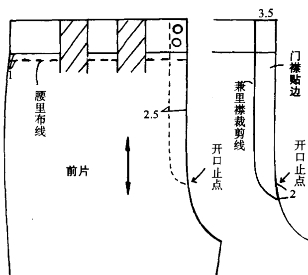
图 3-3 门里襟裁剪图
